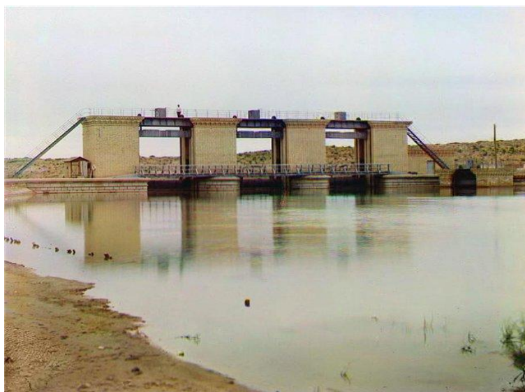
Султанбентская плотина на р. Мургаб.
